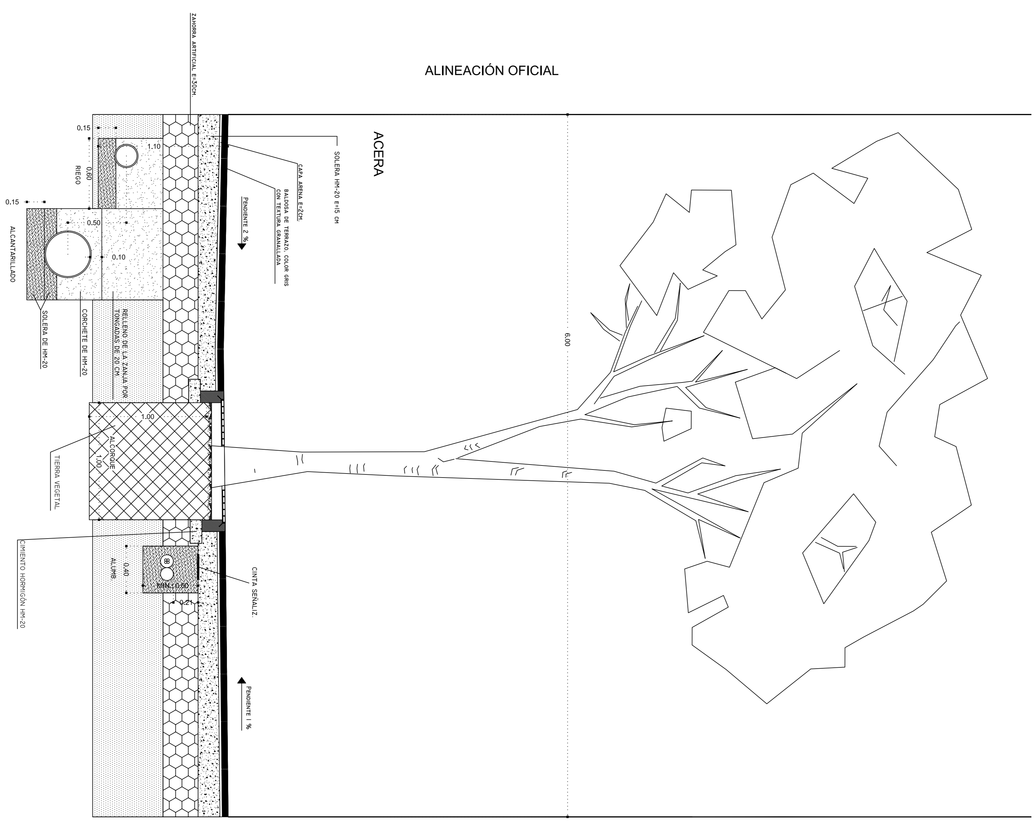
SECCIÓN VP-1
