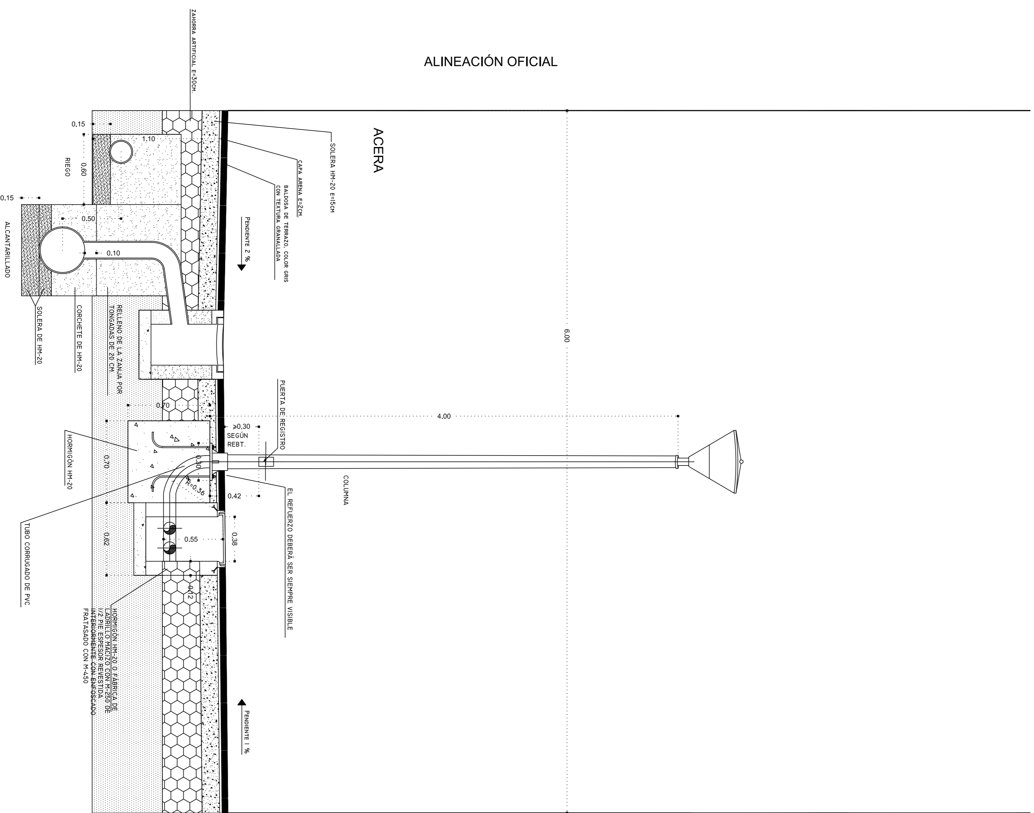
SECCIÓN VP-1
